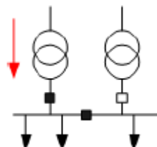
Figure 4.4: Mise hors tension d'un transformateur de réserve
