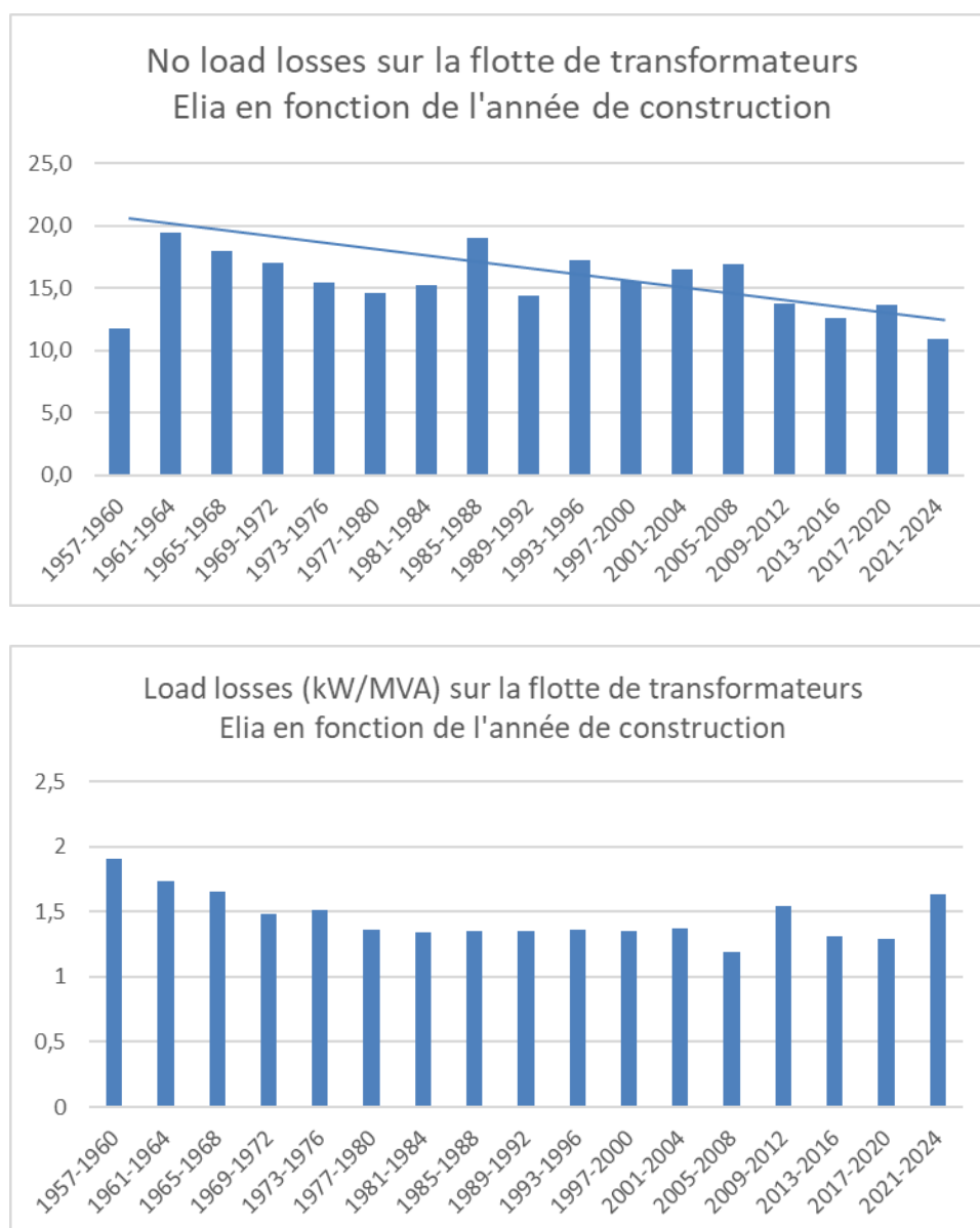
Figure 4.6: Pertes des transformateurs
